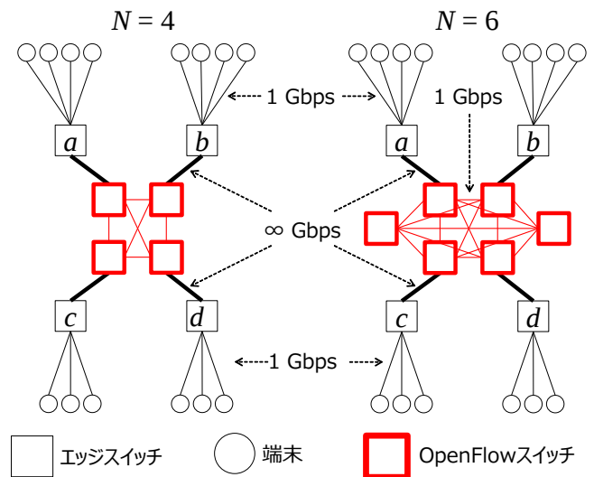
図 9 評価トポロジ. N = 4 の場合 (左) と N = 6 の場合 (右)
