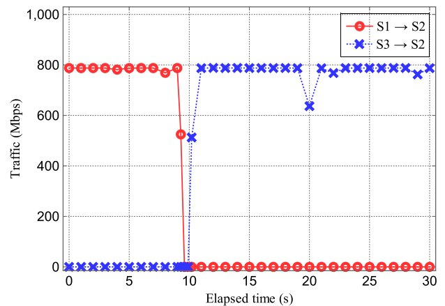
図8 リンクロスト時のトラフィック推移
