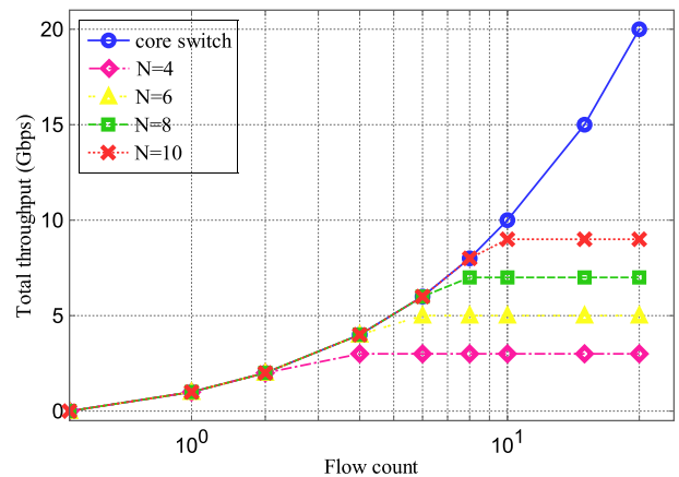
図 10 偏ったフローによる評価
