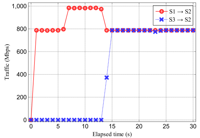
図7 輻輳時のトラフィック推移
