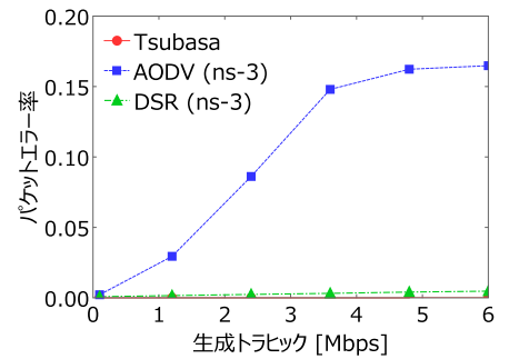
図 11 無線全二重通信の packet エラー率．直線トポロジで 2 ホップ．伝送レートは 6 Mbps．L2 は RFD-MAC．
