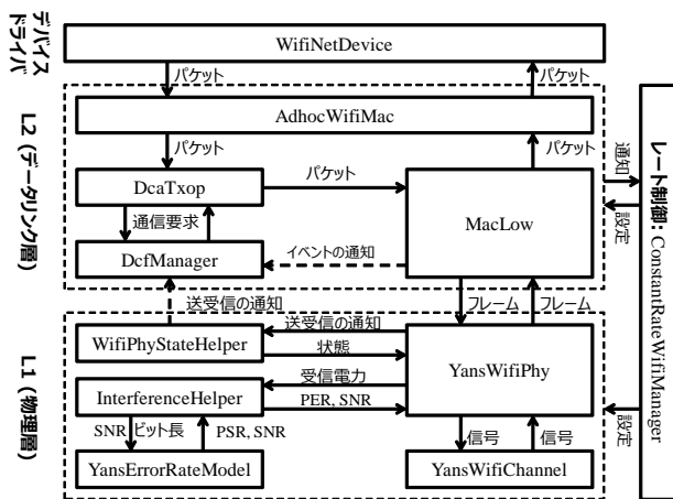
図 7 wifi モジュールの全体像
