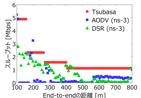
図 15 全二重通信において，10 ノードの直線トポロジでの end-to-end の距離を変えた場合のスループット
