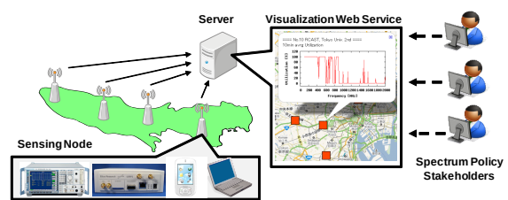
図 5 分散スペクトラムセンシング
